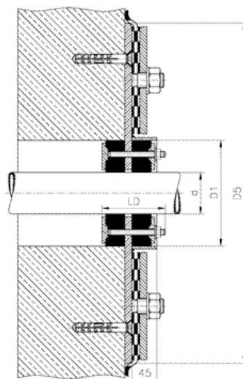
Curaflex Dichtungseinsatz C/2/SD/6 © DÖYNER GmbH & Co
