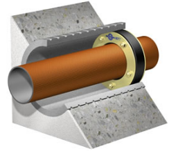
Curaflex 3100-as típusú átvezetés
